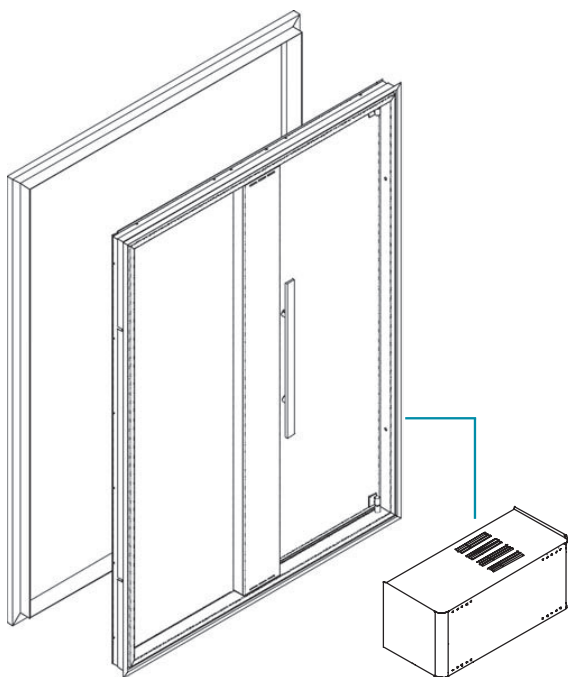
Deur rechts van de zuil handgreep links aanzicht vanaf buitenkant hammam
