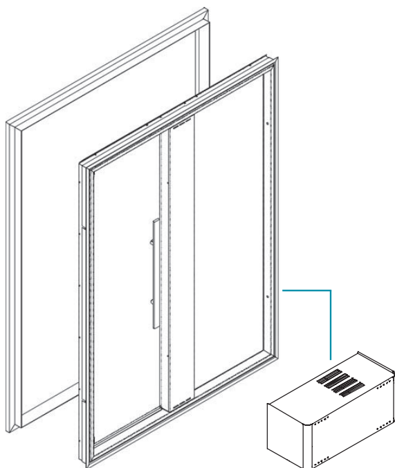
Deur links van de zuil handgreep rechts aanzicht vanaf buitenkant hammam
